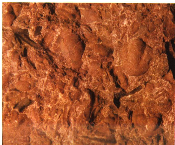
馒头山中寒武統徐庄組三叶虫
