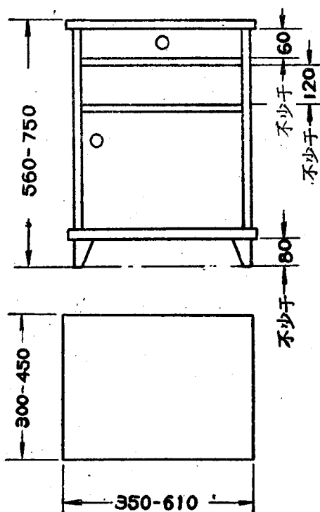
抽屜凹龕单門式
