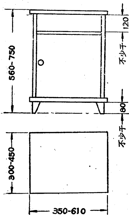
凹龕和单門式
