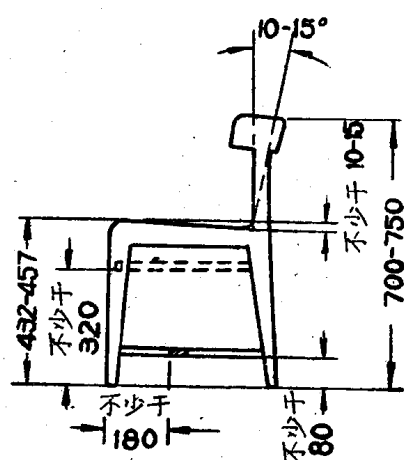
低背小椅剖面圖
