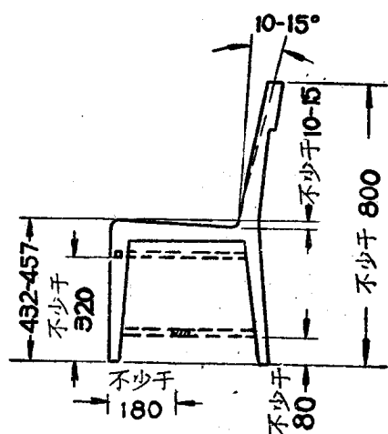
高背小椅剖面圖
