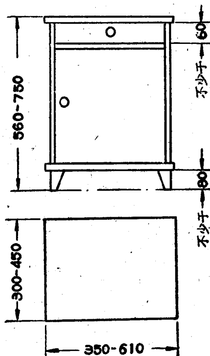
抽屜和单門式
