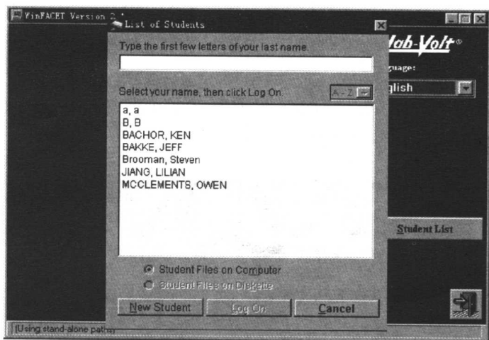
图 1-3 WinFACET 主界面
