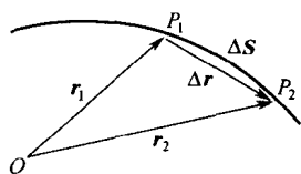
图 1-7 位矢
