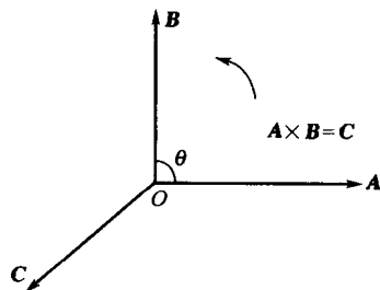
图 1-5 矢量的叉积
