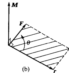
图 1-6 力矩的方向
