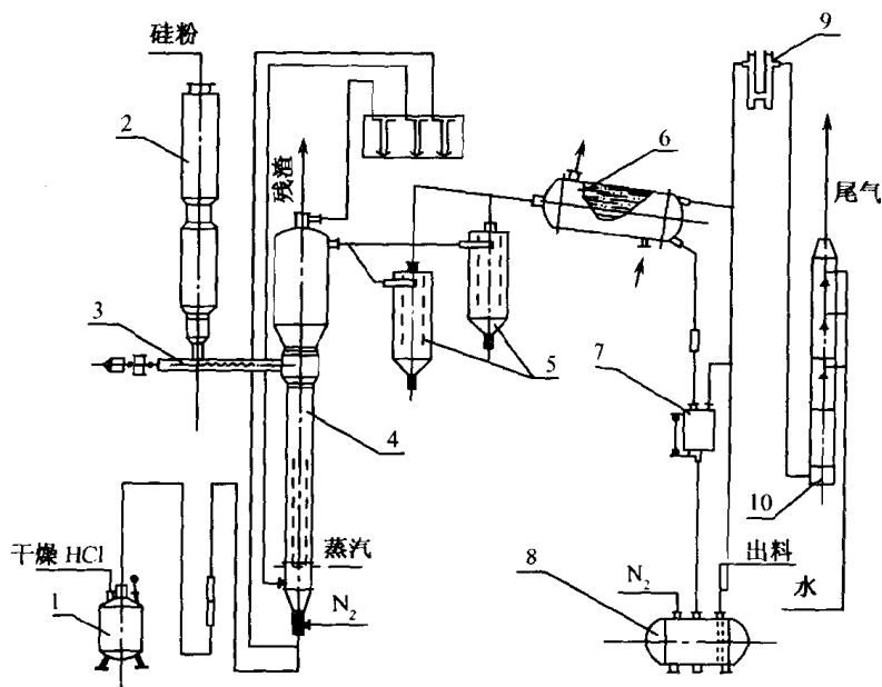
图 1-1 三氯氢硅合成工艺流程
