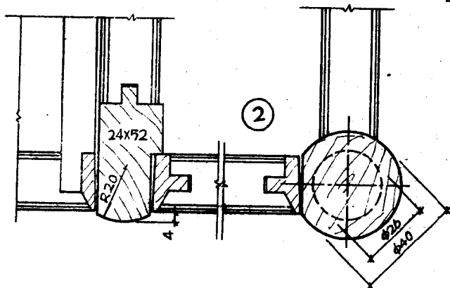
俯视图—C剖视
