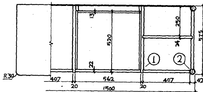
俯视图—B 剖视
