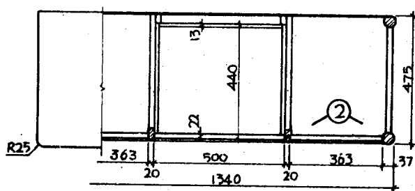
俯视图—C剖视
