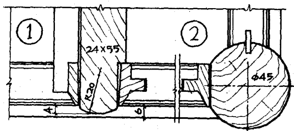
俯视图—B 剖视
