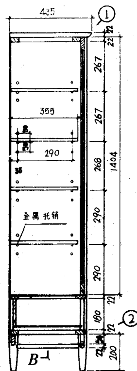
A剖视
