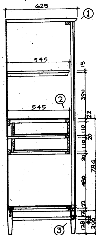
A剖视
