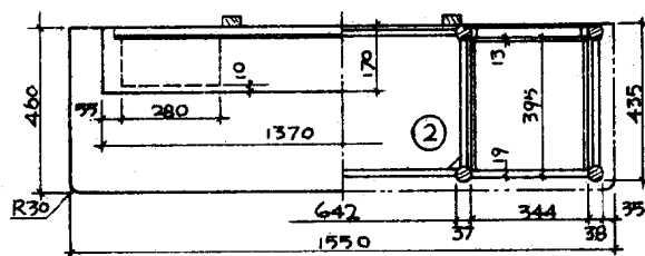
俯视图
