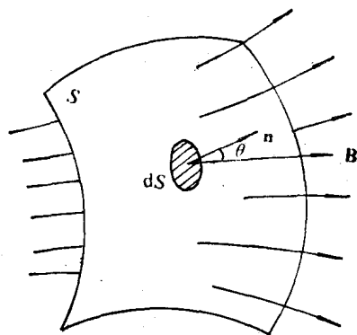
图 11-2 磁通量
