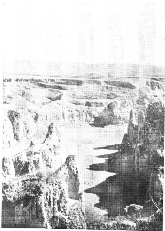
照片 8. 晋西 为冲沟切割的 破碎黄土塬 (山西)
