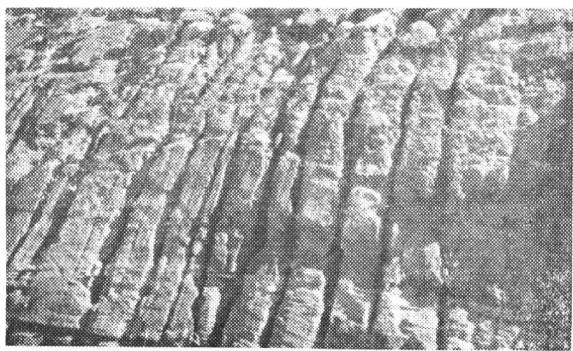
照片 20. 黄土細溝（河北）
