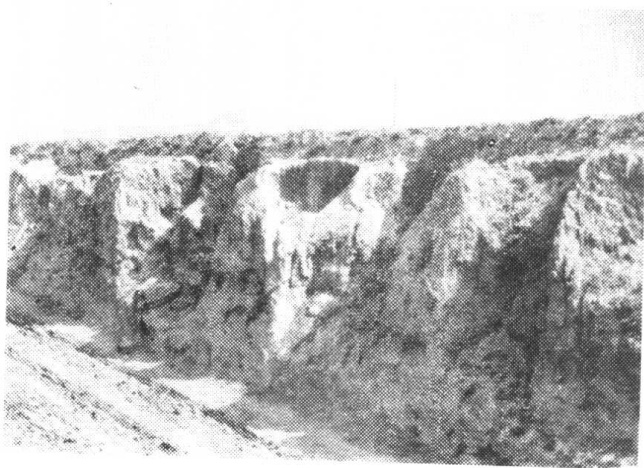
照片 24b. 黄土漏斗状陷穴(河北)
