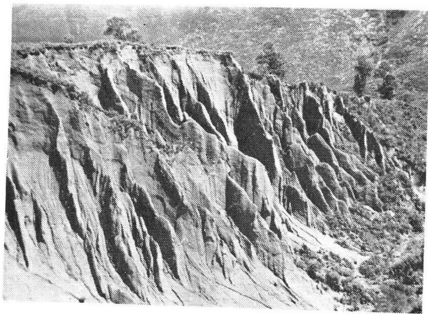
照片 17c. 黄土懸溝 (甘肅)
