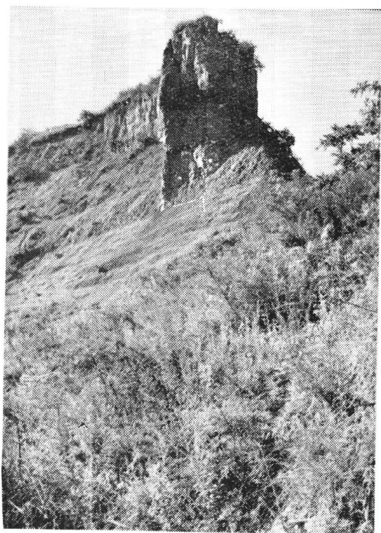
照片 11. 溝間的黃土牆 (甘肅)
