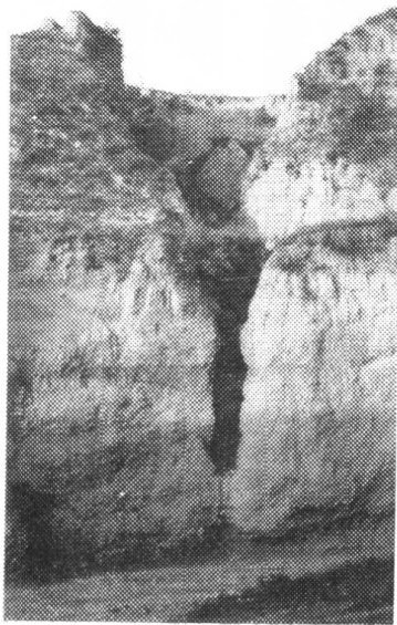
照片 24a. 黄土漏斗状陷穴(河北)
