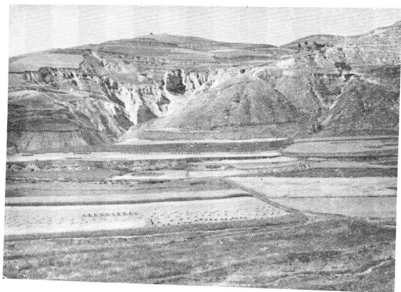
照片 13. 黄土楔溝(甘肅)
