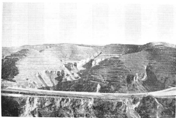
照片 7. 隴东的黃土高原
