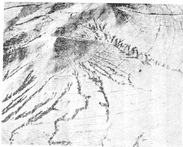
照片 19. 黄土紋溝(山西)
