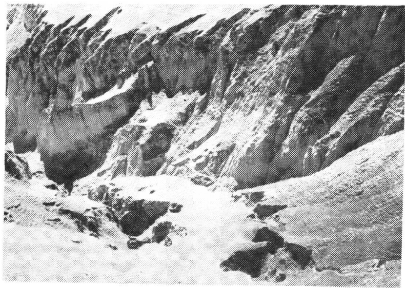
照片 27. 黄土陷溝（甘肅）
