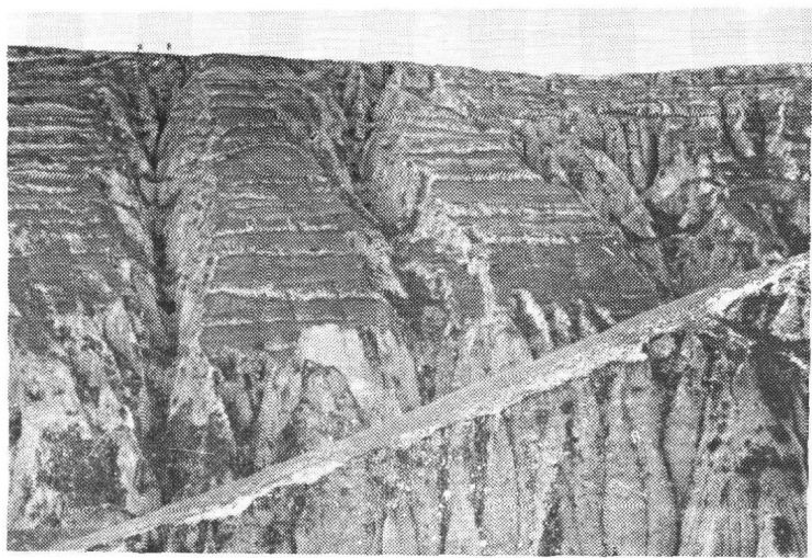
照片 22. 黄土切溝 (甘肅)
