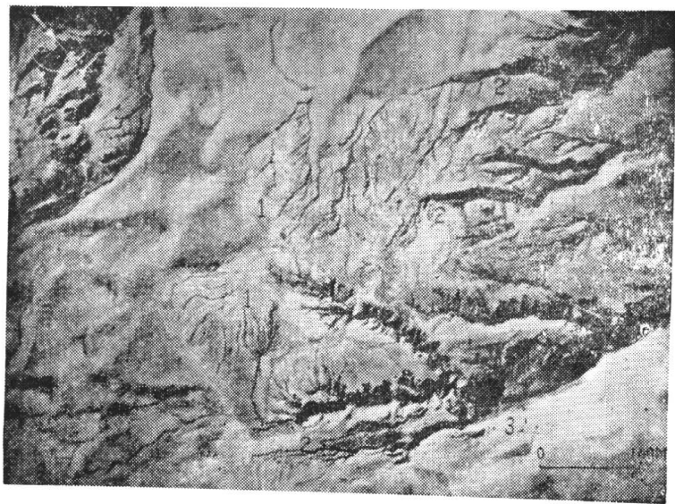
照片 4. 黄土高原鳥瞰
