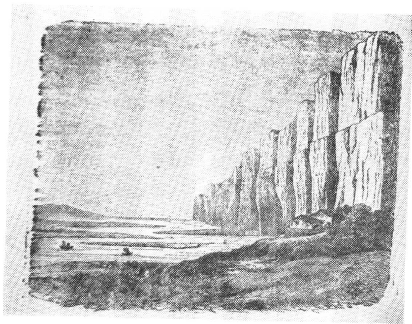
照片 2. 黄河河岸的黄土崖壁 (河南)
