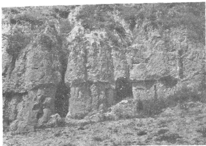
照片 25. 黄土漏斗状陷穴在沟边之出水洞( 陕西 )
