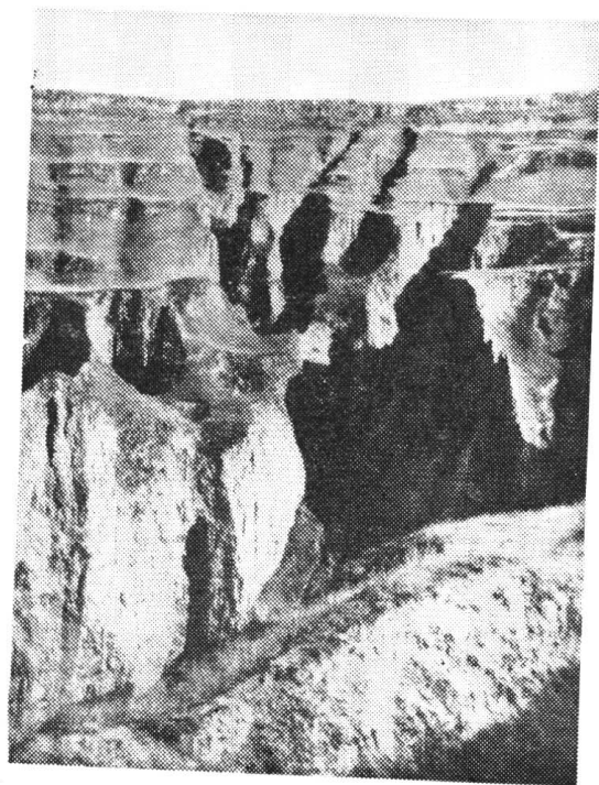
照片 28a. 黄土坡面上的串珠状陷穴(山西)
