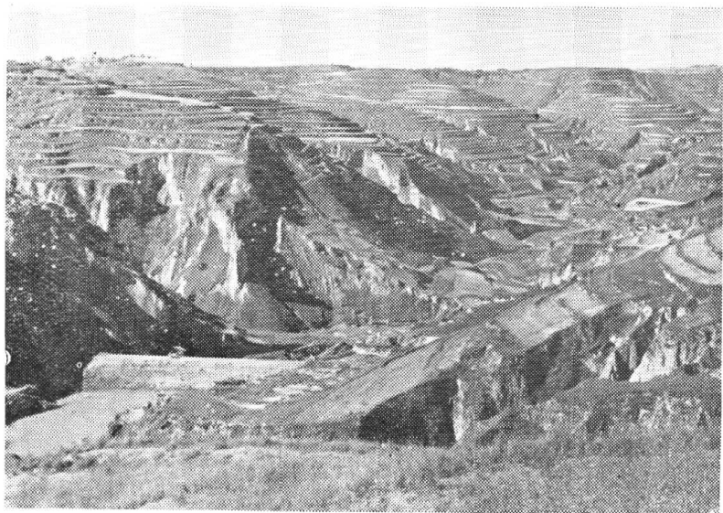
照片 14. 黃土寬溝(甘肅)
