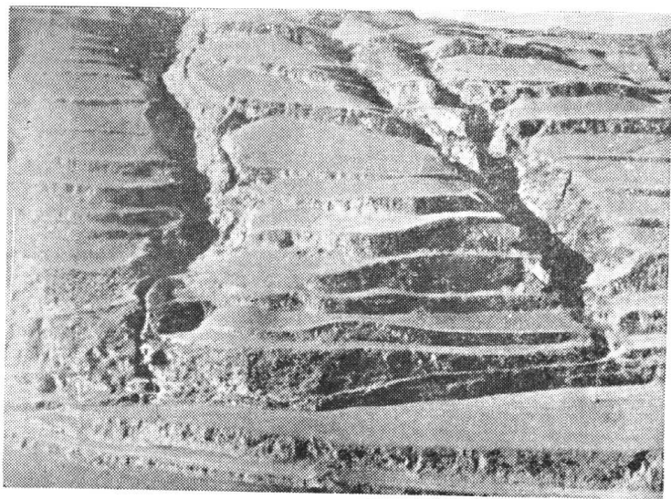
照片 21. 黄土淺溝
