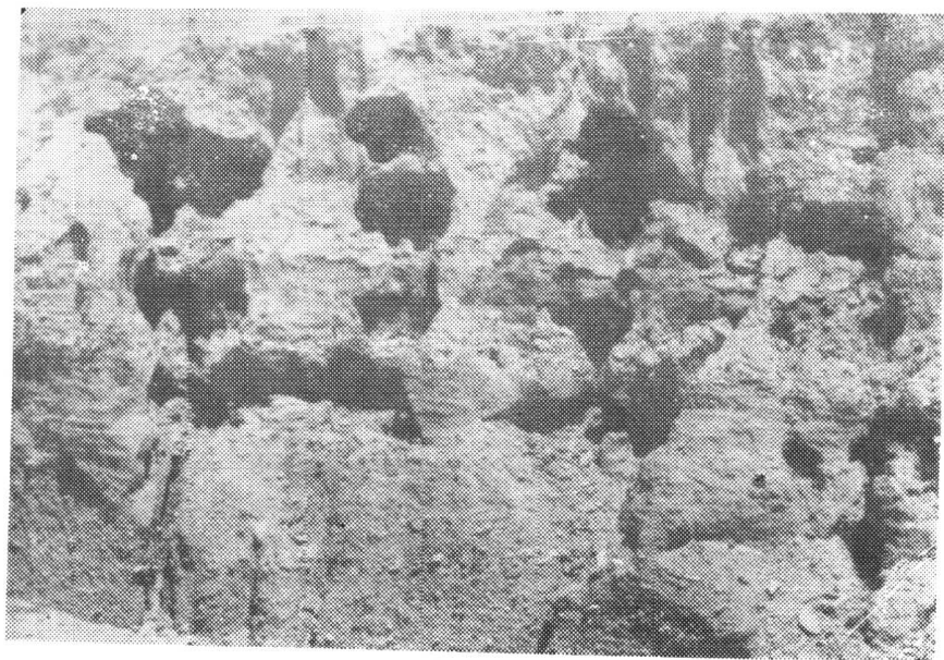
照片 28a. 黄土坡面上的串珠状陷穴(山西)
