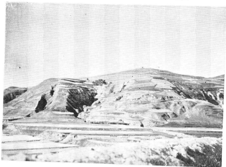
照片 9. 隴中的黄土梁
