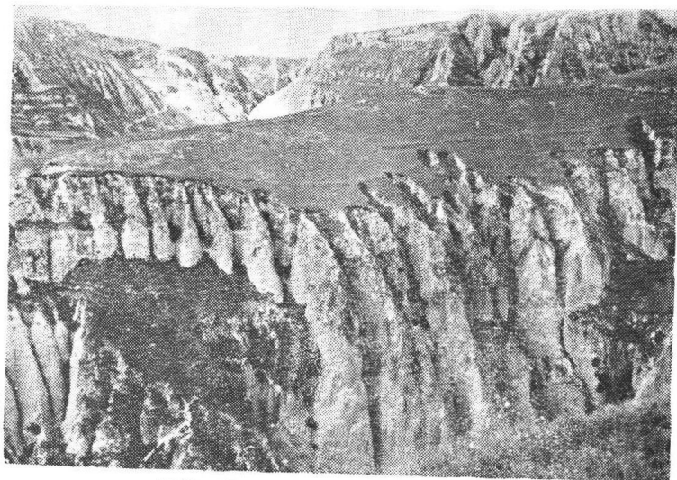
照片 17 a. 黃土雛形懸溝（甘肅）
