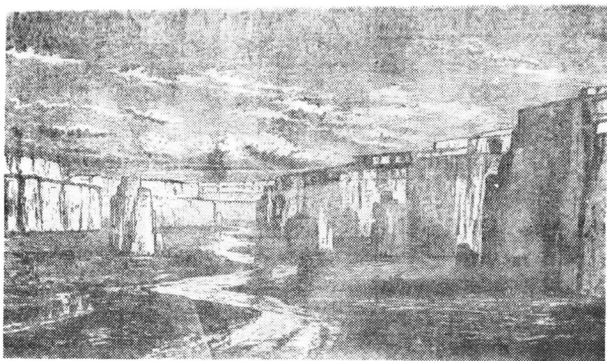
照片 5. 山西太原北方城寨狀黃土景观
