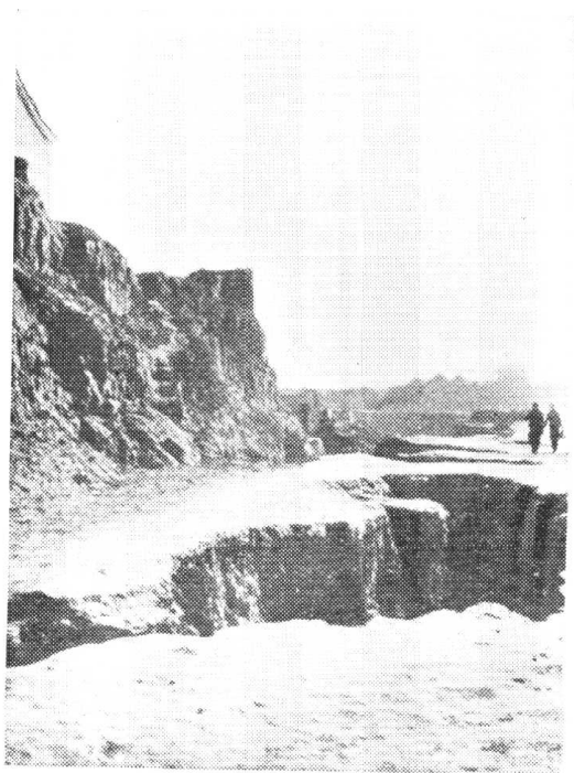
照片 14. 黃土寬溝(甘肅)
