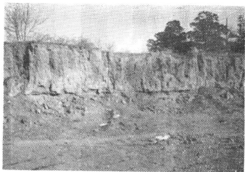
照片 5. 山西太原北方城寨狀黃土景观
