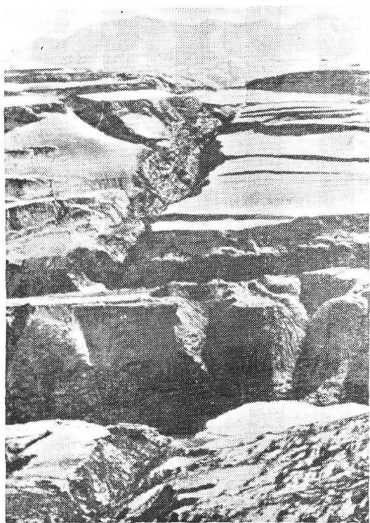
照片 16。黃土急溝
