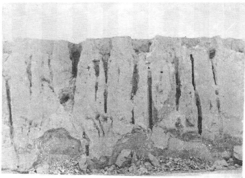
照片 17b. 黄土懸溝 (山西)
