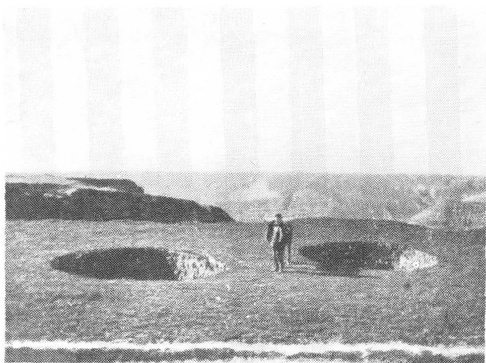
照片 26. 黄土竖井状陷穴
