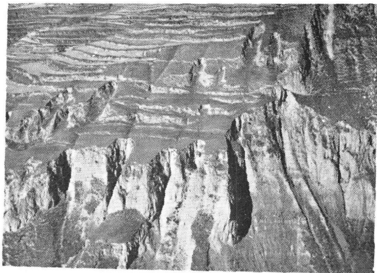
照片 23. 黄土匙形溝 (甘肅)
