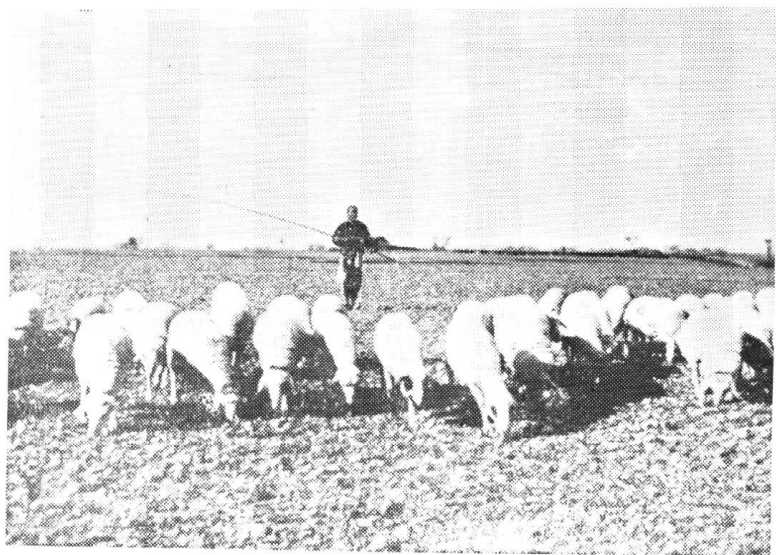
照片 3. 平整如桌面的黄土高原
