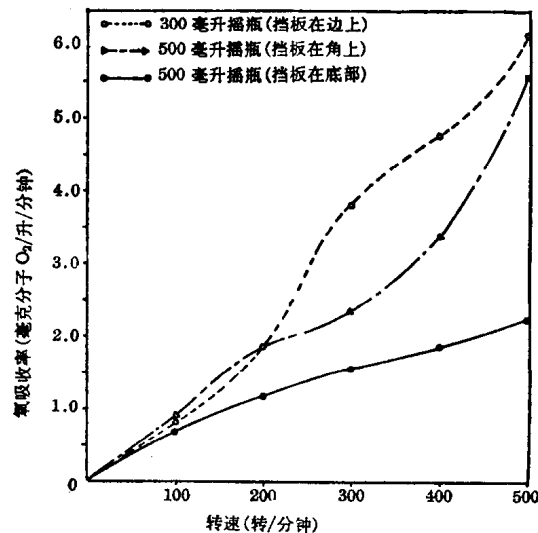
图 3 转速与挡板的位置对氧吸收率的影响
