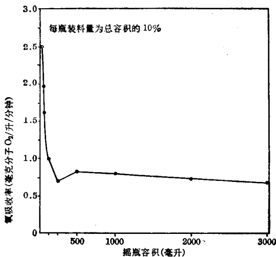
图 4 摇瓶的大小对氧吸收率的影响
