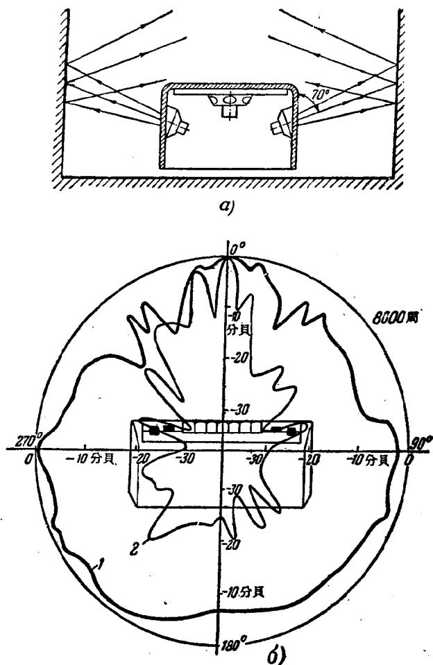
圖 9 可造成立体声效应的发声系统的辐射方向图，以及喇叭在收音机壳内的布置。
