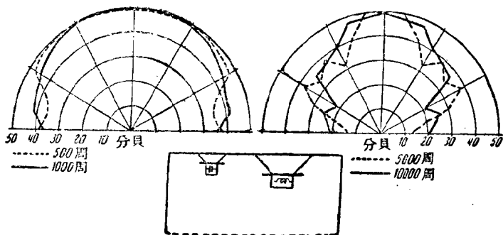
圖 8 两只不同型式喇叭在收音机机壳內的布置以及这种发声系統的輻射方向圖。
