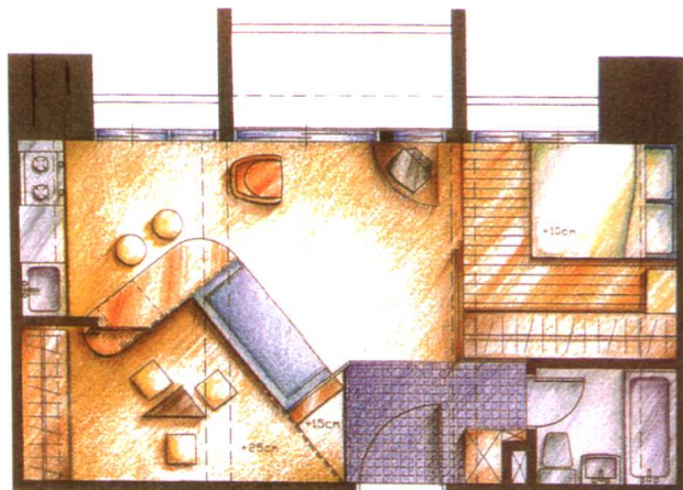
设计后的平面配置图
