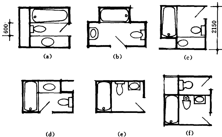
图1-1-1 卫生洁具布置不当的例子
