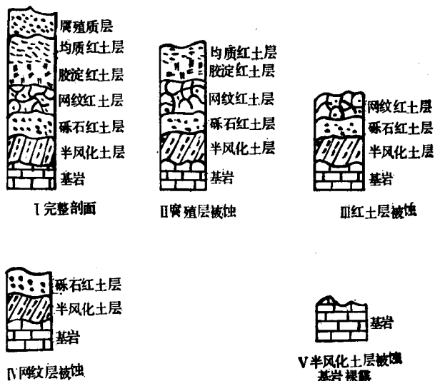
图1 低丘红壤 (第四纪红土母质) 剖面构型
