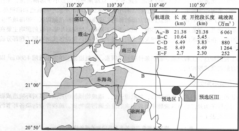
图 1-1 航道疏浚工程示意图 (图中：粗线段为需疏浚航道段，细线段为不需疏浚航道段)
