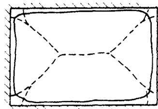
(d) Yield line mechanism-Stage C
