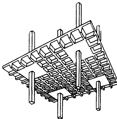
(b) Waffle slab
