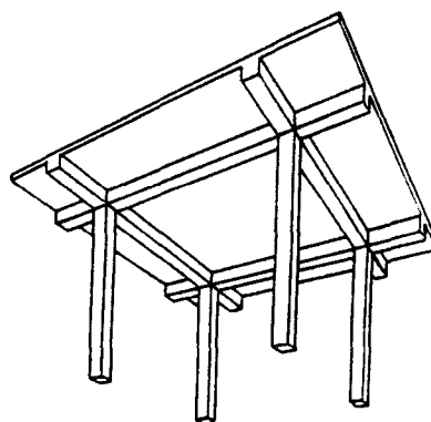
(d) Two-way slab with beams
