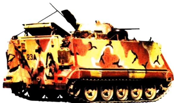
美国 M113 履带式装甲人员运输车
