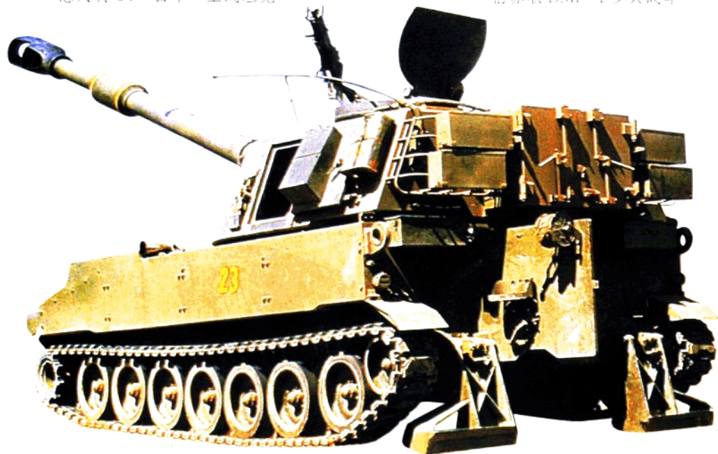
美国 M109A5 自行榴弹炮
