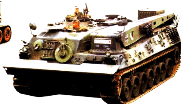
德国 BP2-2A2 装甲抢救车
