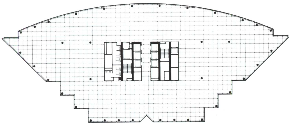
底层平面
