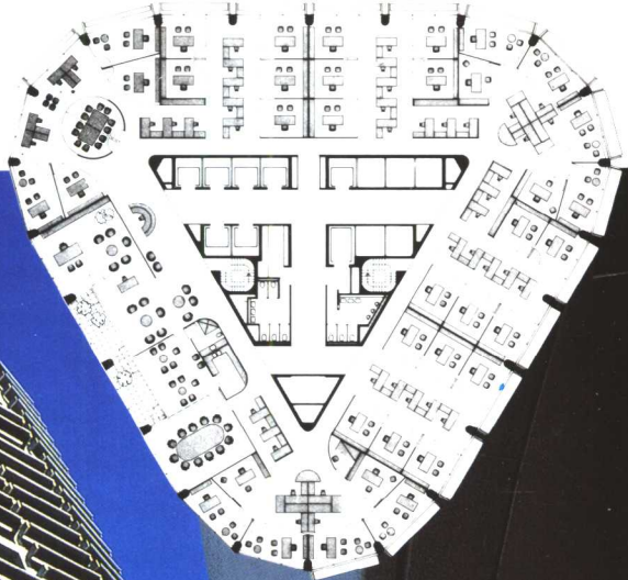
标准层平面
