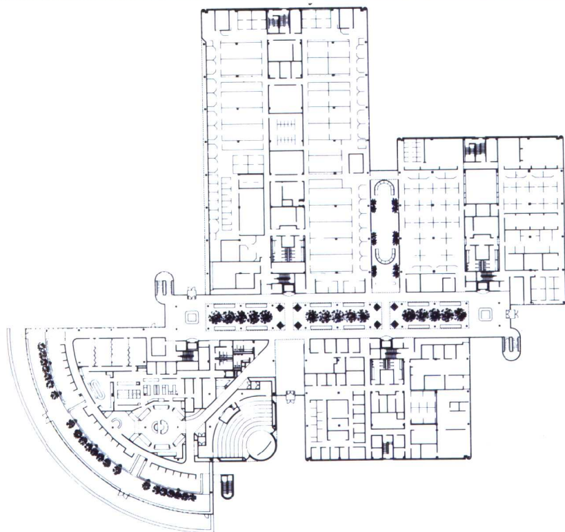
(上图) 首层平面
