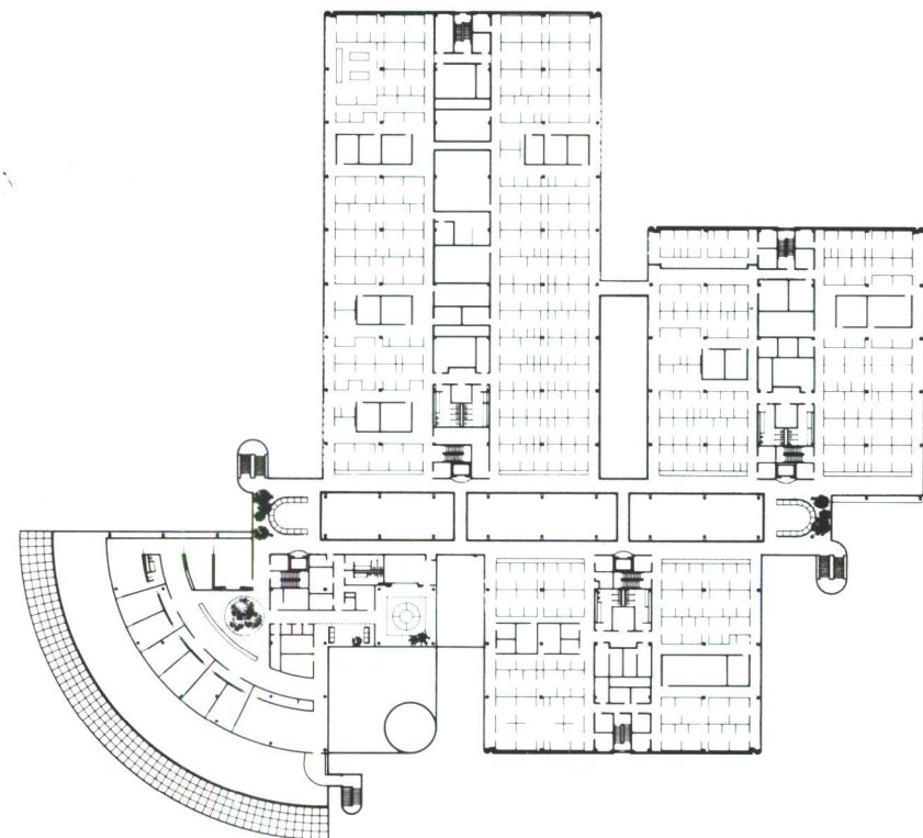
(上图) 三层平面
