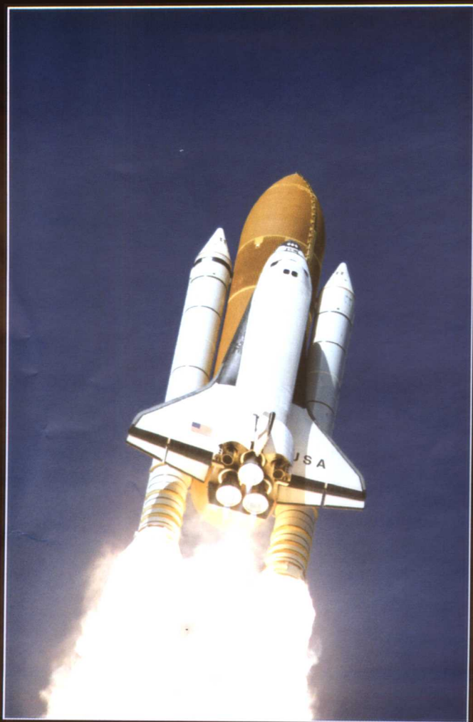
为了探求宇宙的真相，人类向太空发射了众多的卫星、宇宙探测器和宇宙飞船。上图是腾空而起的美国 USA 宇宙飞船。
