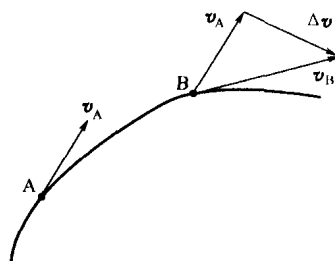
图 1-3 速度增量
