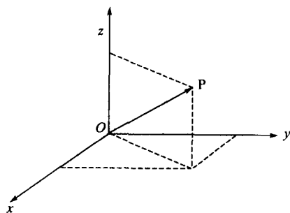
图 1-1 位矢
