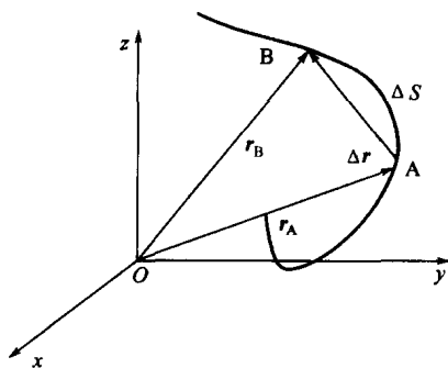
图 1-2 位移
