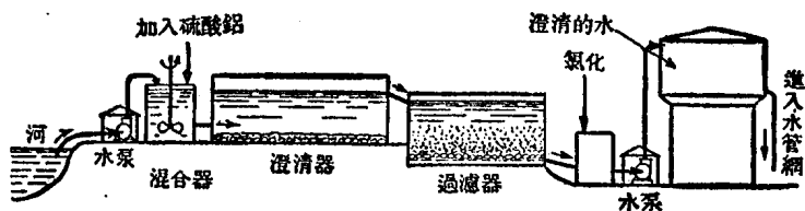
圖 2 河水澄清圖解。
