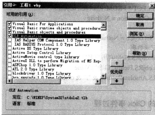
图 1-10 “引用”对话框
