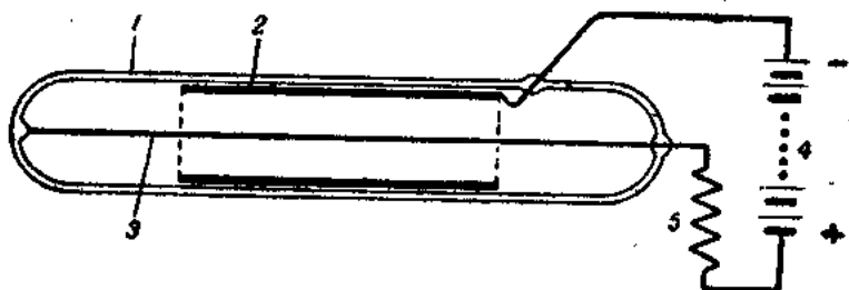
圖3. 蓋格-密勒計數器的略圖；1—玻璃圓筒；2—陰極（金屬圓筒）； 3—陽極（金屬細線）；4—高壓電池組；5—高電阻。
