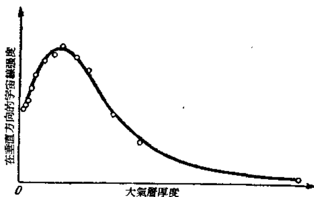
圖 2. 在垂直方向的宇宙線強度隨高度的變化
