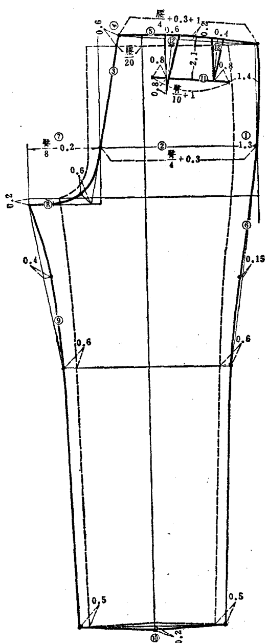
图3 后片轮廓线图
