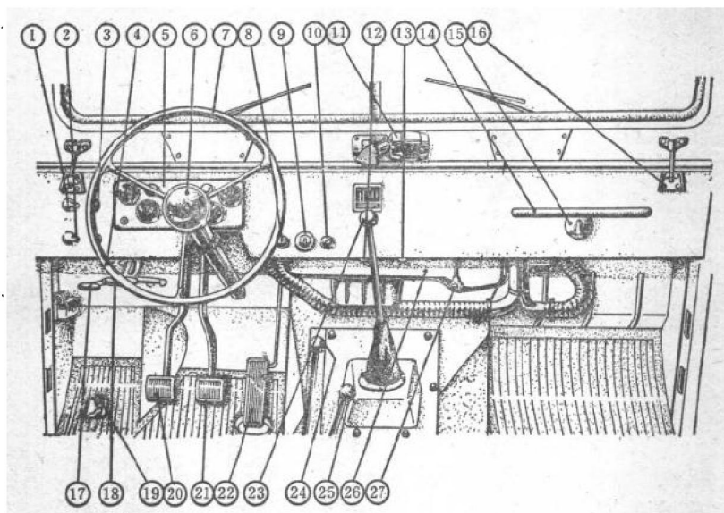
图1 驾驶操纵机构和仪表的布置
