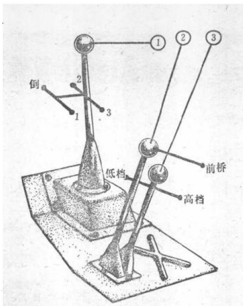
图2 变速器和分动器操纵杆的布置
