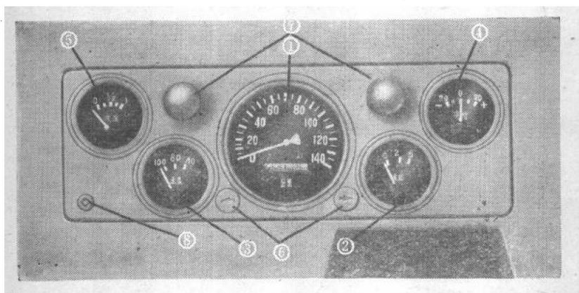
图3 综合仪表板总成
