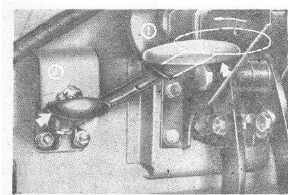
图13 手制动手柄和百叶窗控制手柄
