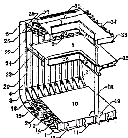
图2-1 钢质干货船体结构布置图（混合结构式）
