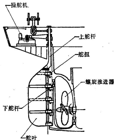
图2-2 螺旋推进器和舵
