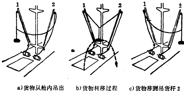
图2-6 双吊杆工作示意图
