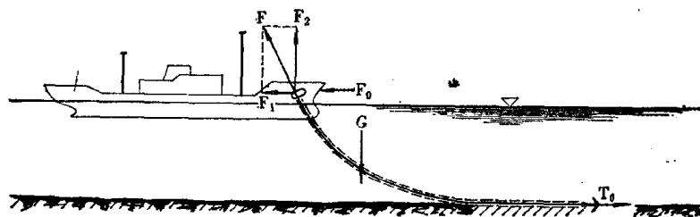
图2-4 锚与锚链的工作
