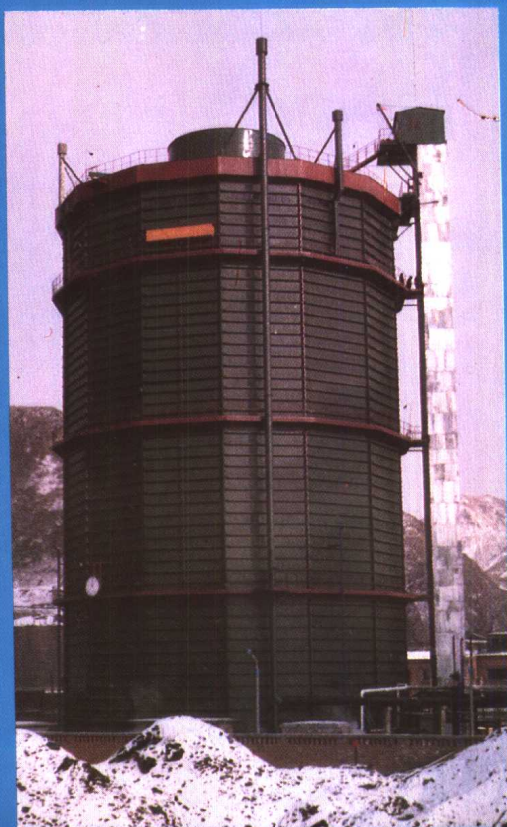
20,000米 3 乾式煤氣櫃
