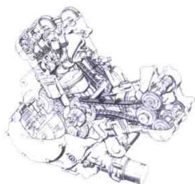
③ 发动机立体剖视图
