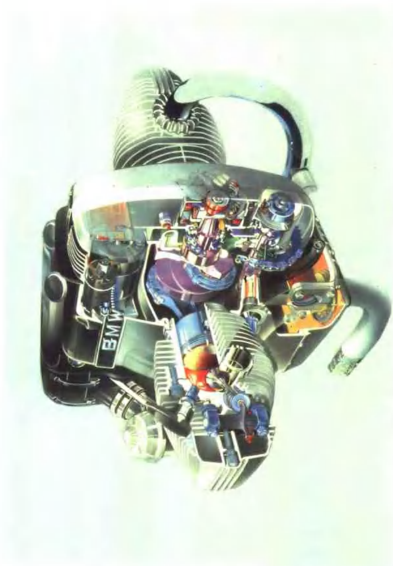
彩图 8 德国 BMW(宝马)公司的发动机剖示图兼工作原理图
