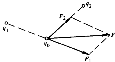
图 11-2-2 电力叠加原理
