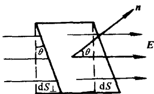
图 11-1-2 通过 dS 的电通量
