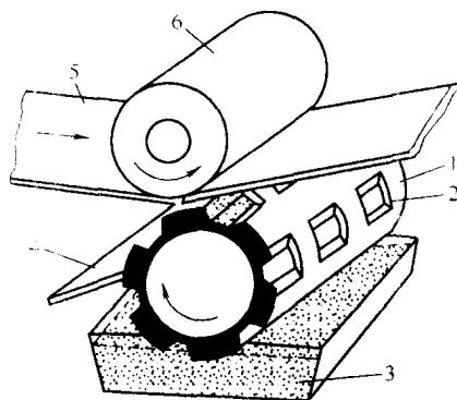
图 1-2 凹版印刷机印刷部的构成 1—印版滚筒；2—图文部分；3—墨斗； 4—刮墨刀；5—纸张；6—压印滚筒
