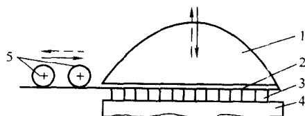
图 1-5 平压平印刷机印刷部的构成 1—压印平板；2—承印物；3—印版； 4—版台；5—着墨辊
