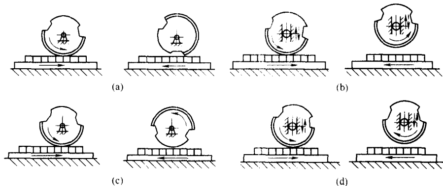
图 1-7 圆压平印刷机的工作原理
