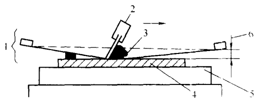
图 1-4 丝网印刷机印刷部的基本构成 1—丝网印版；2—刮墨板；3—油墨；4—承印物； 5—丝网印刷台；6—网版间隔
