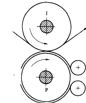
图 1-8 圆压圆印刷机印刷部的构成
