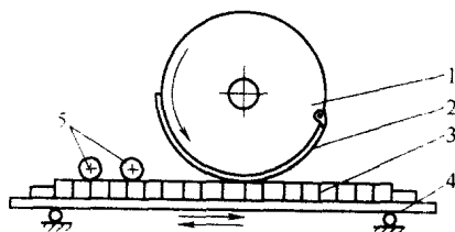
图 1-6 圆压平印刷机印刷部构成示意 1—压印滚筒；2—承印物；3—印版； 4—版台；5—着墨辊
