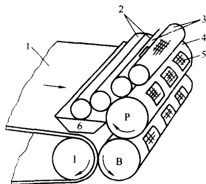
图 1-3 平版印刷机印刷部的构成 1—纸张；2—水辊；3—墨辊；4—空白部分； 5—图文部分；6—水斗； P—印版滚筒；B—橡皮滚筒；I—压印滚筒
