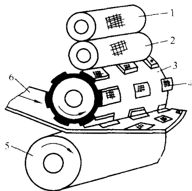
图 1-1 凸版印刷机印刷部的构成 1—匀墨辊；2—着墨辊；3—印版滚筒； 4—印版；5—压印滚筒；6—纸张
