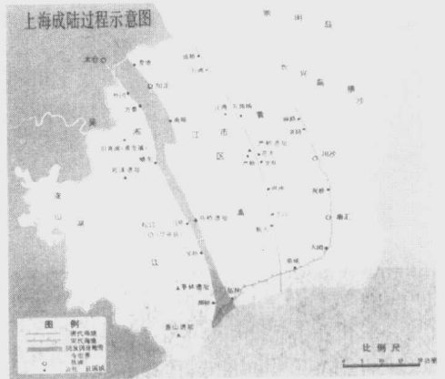
上海成陆过程示意图
