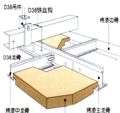
明架式吊装结构图
