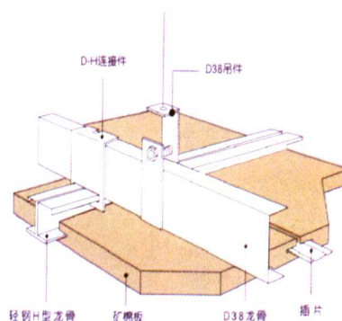
暗插式吊装结构图
