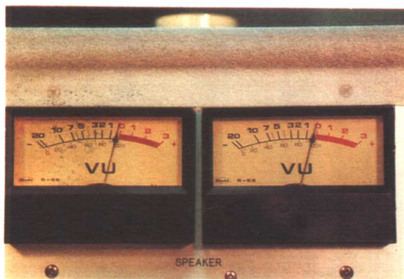
彩图 44 UV 表
