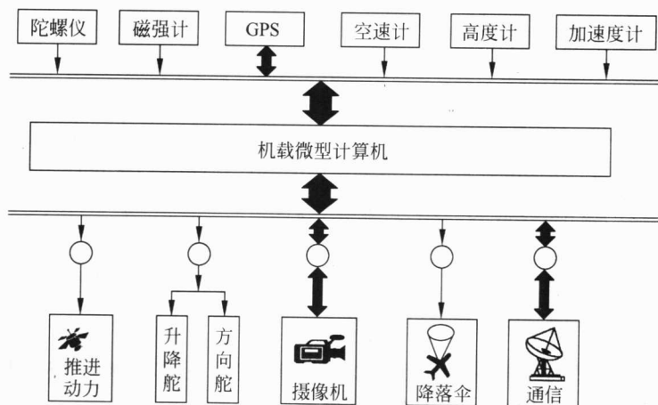
图 1-4 微型飞行器测控组合
