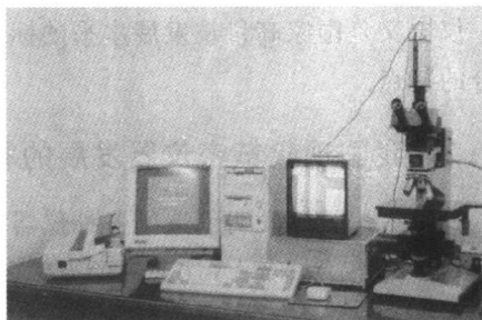
测量分辨率: 0.01 \mu\text{m} 测量精度: \pm 0.05\mu\text{m}
