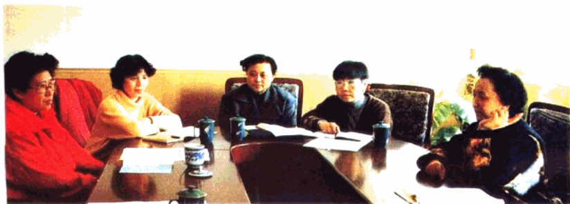
学习理论
