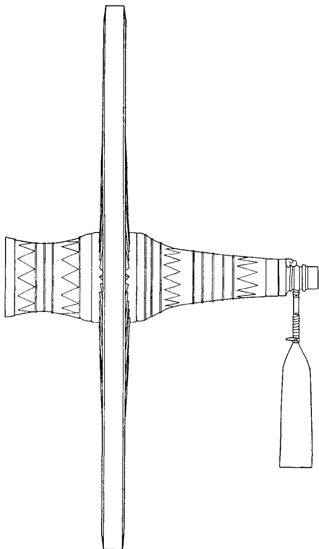
图 1-7 2 号铜车上的轂、舌与飞铃
