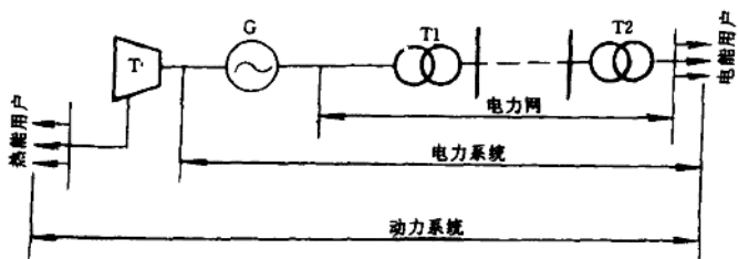
图 2-1 动力系统、电力系统和电力网
