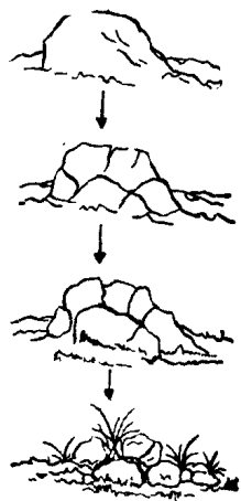
图1—1 岩石的风化过程示意图
