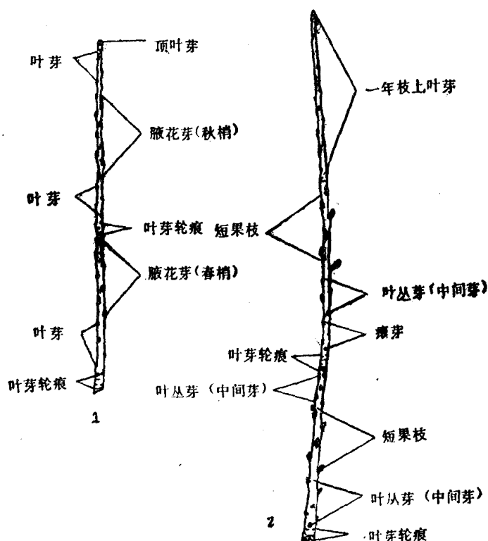
图3 芽的异质性
