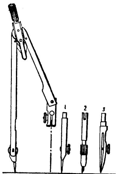
图 1-6 圆规及其附件
