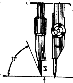
图 1-8 圆规插脚上铅芯的处理
