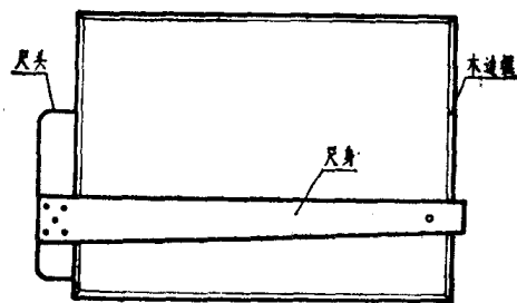
图 1-1 图板与丁字尺
