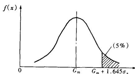
图 2-1 荷载标准值的取值
