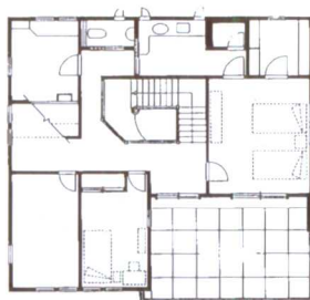
二层平面图
