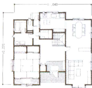
一层平面图
