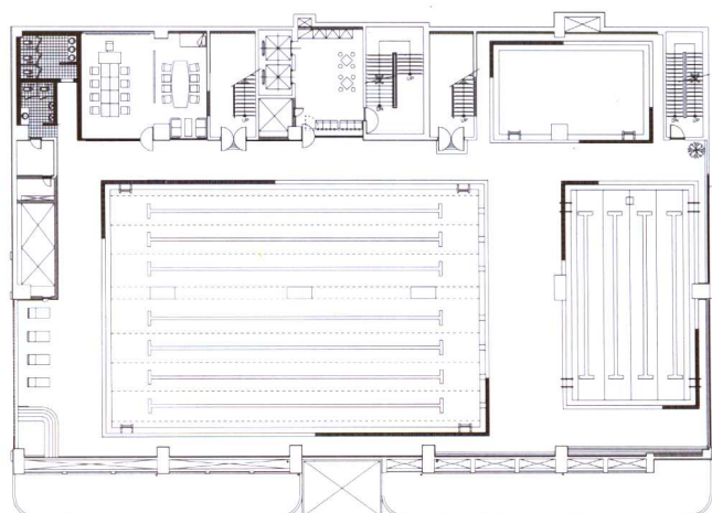
1层平面图
