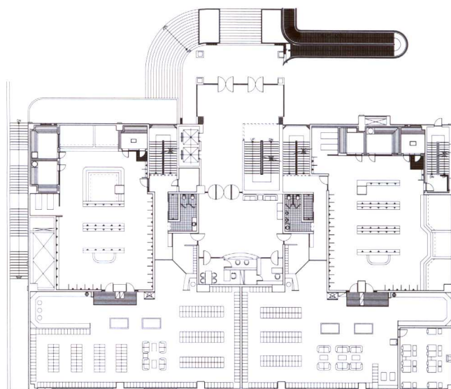
2层平面图
