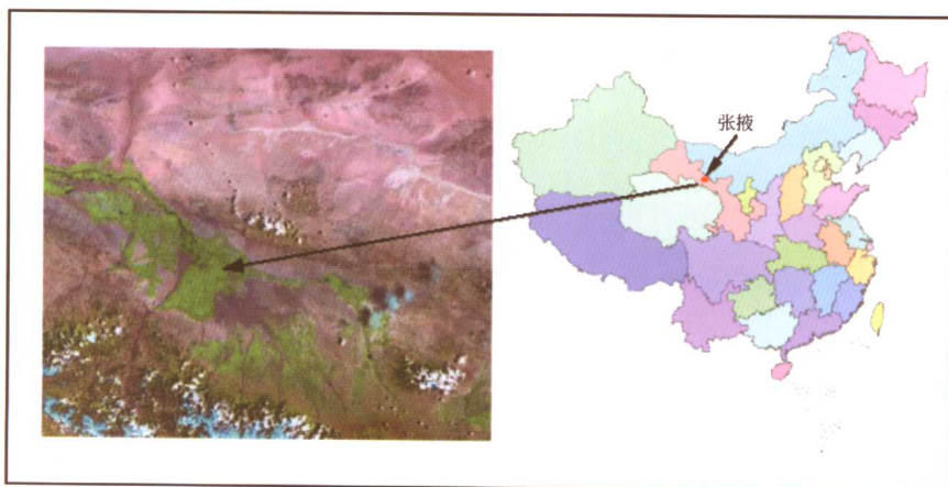
彩图 2 甘肃张掖所在的黑河流域的遥感影像
