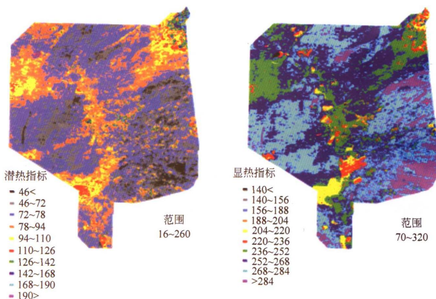
彩图 9 用 CECM 模式计算的美国新墨西哥的 Jornada 地区的潜热和显热指标
