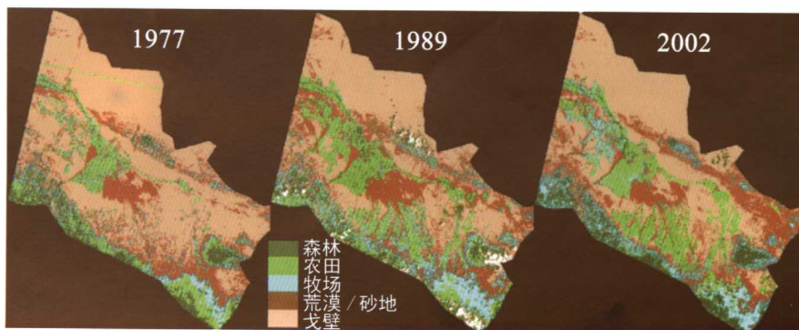
彩图 4 不同时期的土地利用变化
