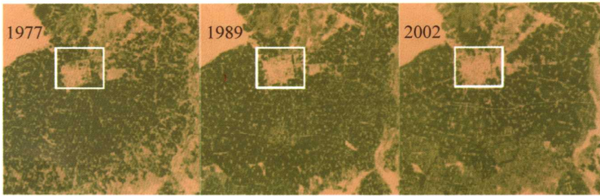
彩图 5 不同时期植被覆盖度的变化
