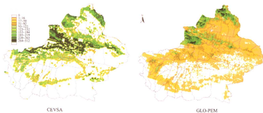
彩图 1 用 GLO-PEM 和 CEVSA 模型估计的新疆 NPP 在 1981—2000 年期间的平均值
