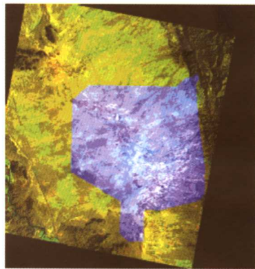
彩图 7 中国新疆阜康和美国新墨西哥的 Jornada 地区的遥感影像
