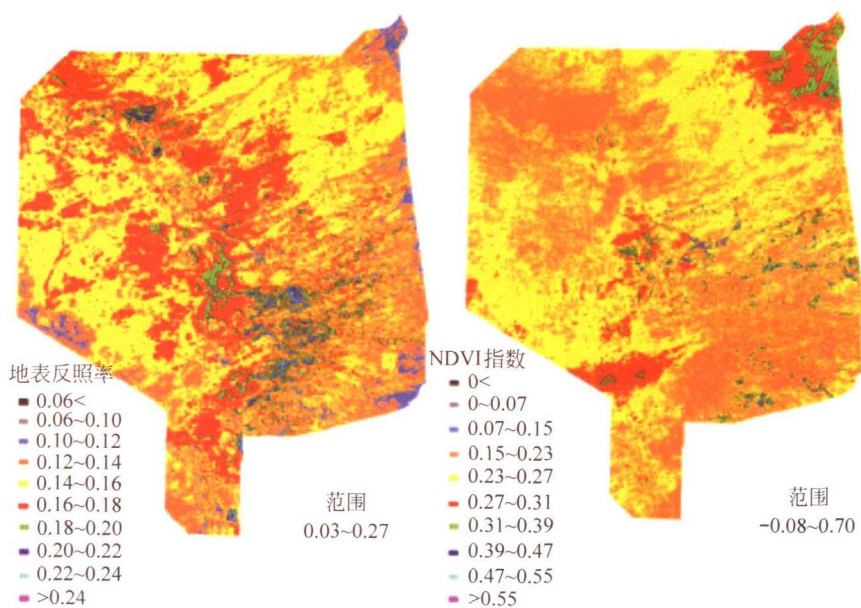
彩图 8 用遥感影像数据计算的美国新墨西哥的 Jornada 地区的地表反照率和 NDVI 指数
