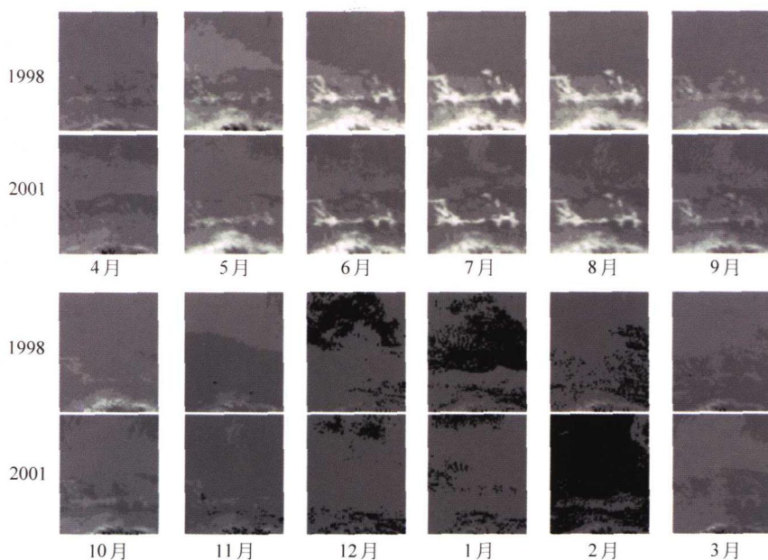
彩图 10 用遥感影像数据计算的中国新疆阜康地区的 2 年 12 个 NDVI 指数
