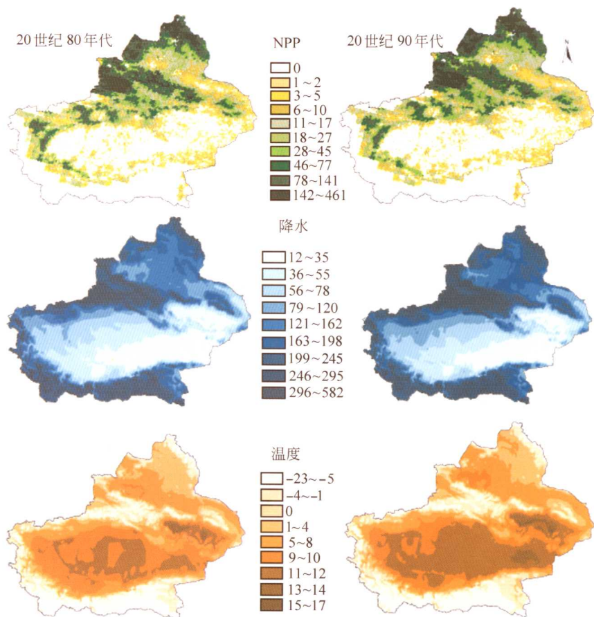
彩图 3 新疆在 1981—2000 年期间的 NPP、温度和降水变化
