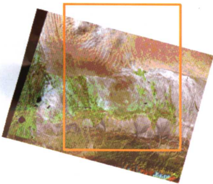
彩图 7 中国新疆阜康和美国新墨西哥的 Jornada 地区的遥感影像
