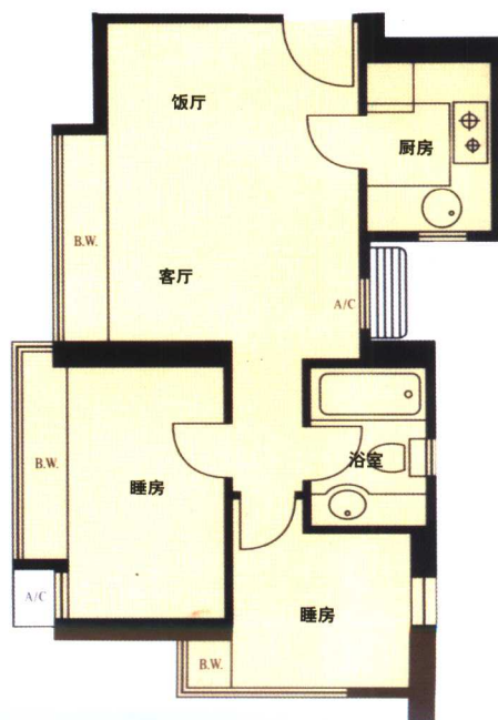
平面设计图
