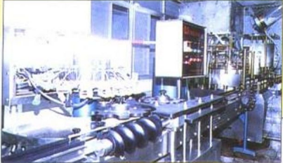
密封式灌装线
