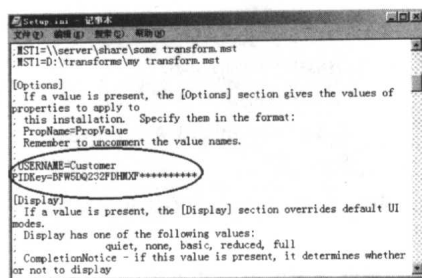
◆这样就可以让 Office XP 帮你自动输入 CDKey
