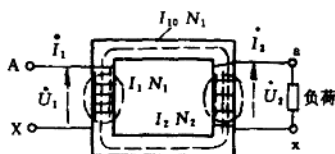
图 1-2 配电变压器原理图
