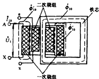
图 1-1 配电变压器的磁路
