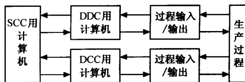
图 1-6 监督计算机控制系统框图
