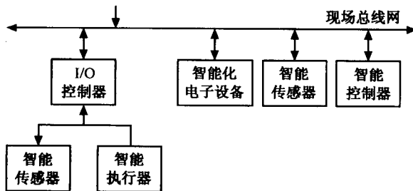
图 1-8 现场总线控制系统的组成
