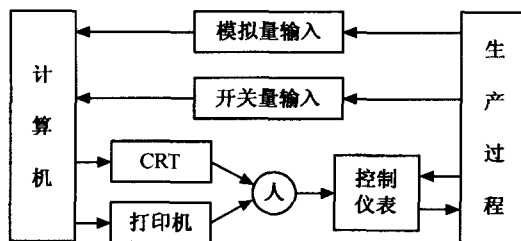
图 1-4 操作指导控制系统框图
