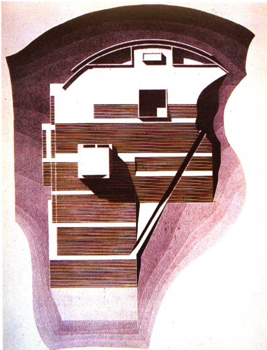
图1 飞鸟历史博物馆总平面布局
