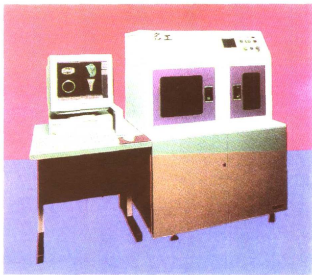
与CAD系统相联接的“名工”激光造型系统
